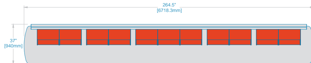
LINEAR C-TOP EDGE DETAIL
