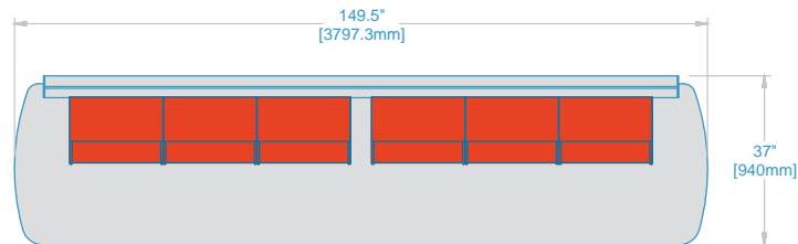
LINEAR C-TOP EDGE DETAIL
