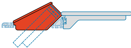
2RU TURRET
