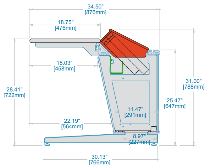
2RU TURRET
